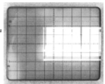
Figure 3 MODE : "del" (DELAY = retarder) TIME/DIV. : 5 ms/cm Couplage de déclenchement:TV-F Front de déclenchement : descendant (-) Temps de retard : 4 cm x 5 ms = 20 ms
