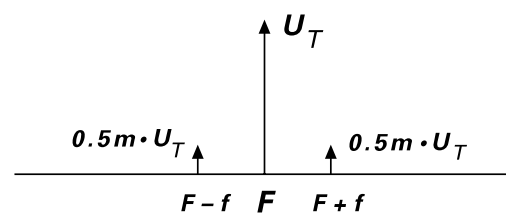
Fig. 1 Spectre de modulation d'amplitude (m=50%).
