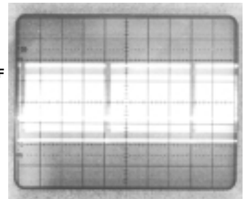
Figure 2 MODE : "sea" (SEARCH=rechercher) TIME/DIV. : 5 ms/cm Couplage de déclenchement:TV-F Front de déclenchement: descendant (-) Temps de retard : 4 cm x 5 ms = 20 ms
