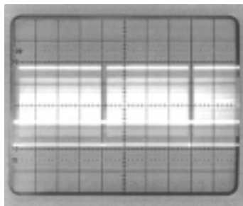
Figure 1 (signal vidéocomposite) MODE : DEL.MODE OFF TIME/DIV : 5 ms/cm Couplage de déclenchement : TV-F Front de déclenchement : descendant (-)
